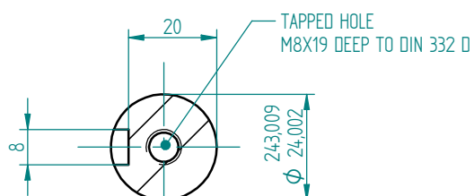
Przekrój A-A 1:1
